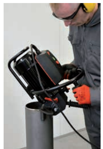
Biselado de tubo (opcional)
